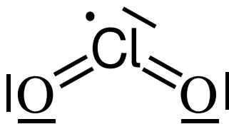
Chlordioxid ( \text{ClO}_2 )
